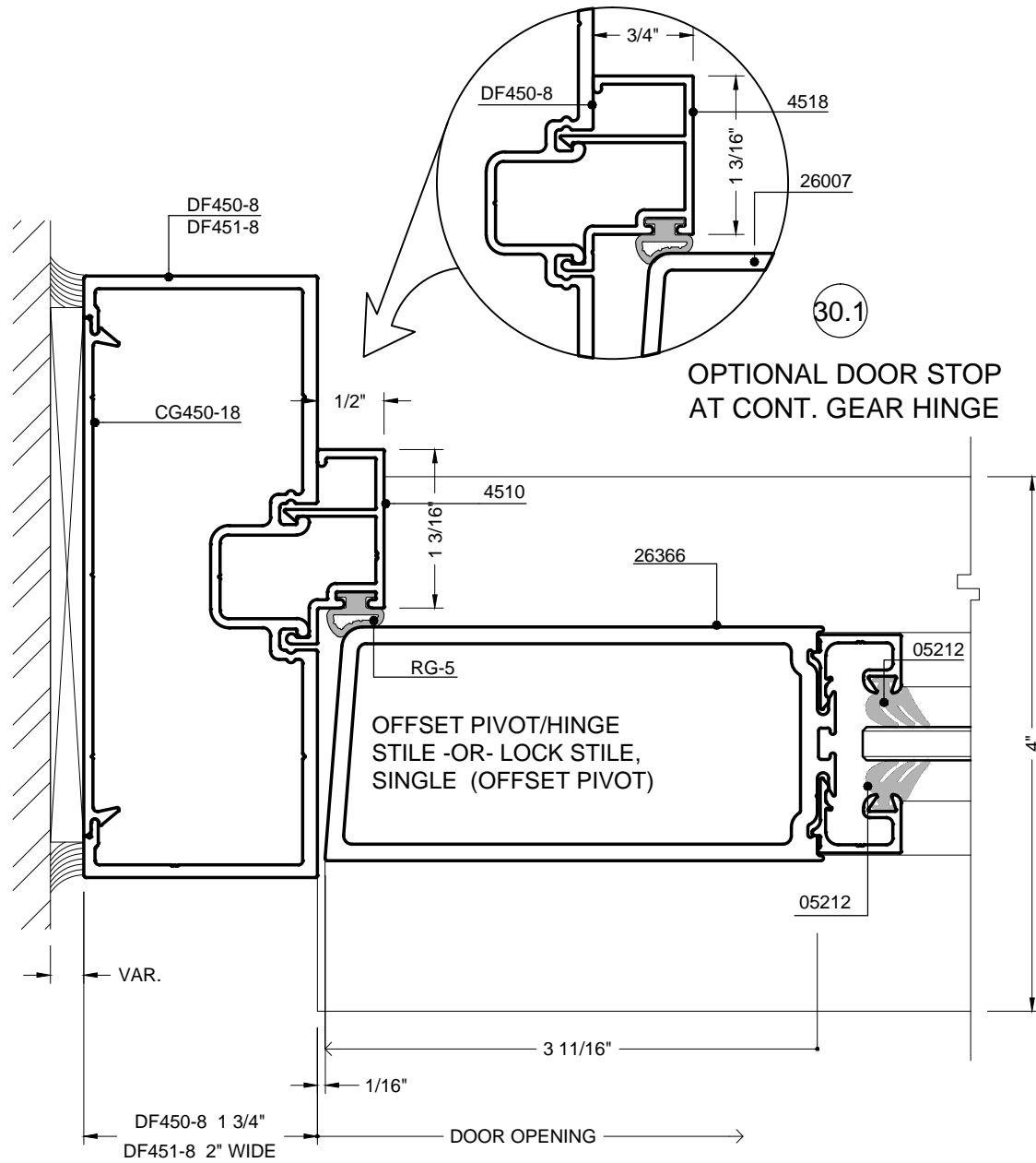
30 MS DOOR JAMB (STANDARD) OFFSET PIVOT & BUTT HINGE
