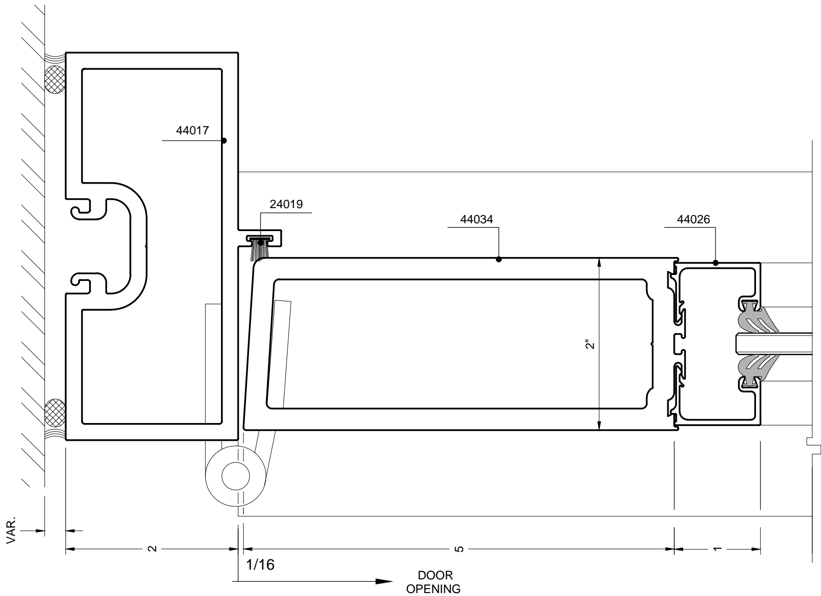
50 DOOR JAMB (STANDARD) OFFSET PIVOT & BUTT HINGE
