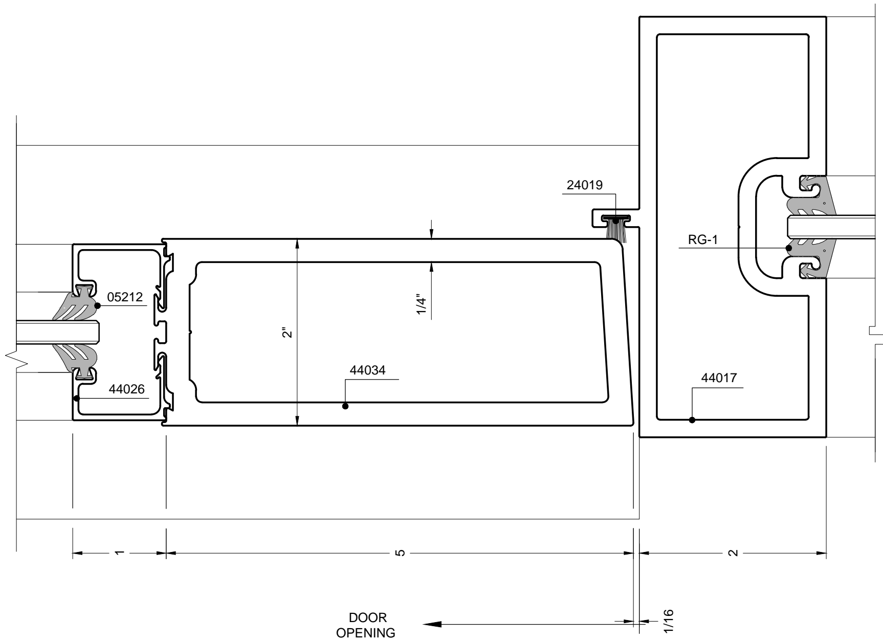
(52B) DOOR JAMB - LOCK STILE
