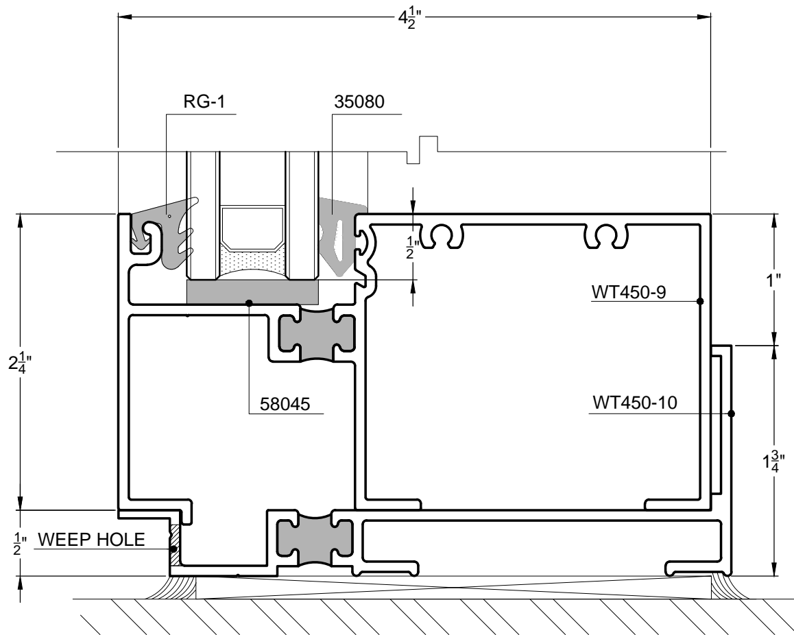
(12A) SILL
