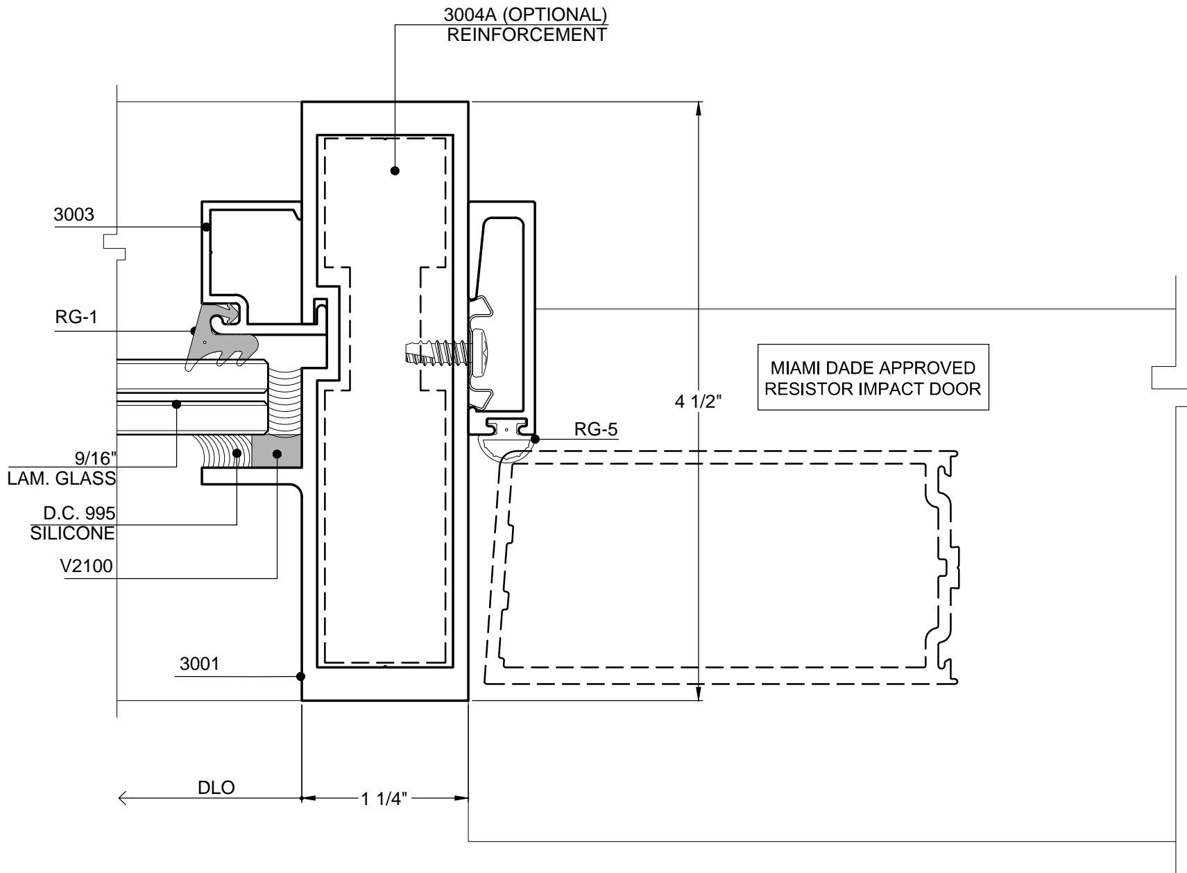
40 DOOR JAMB
