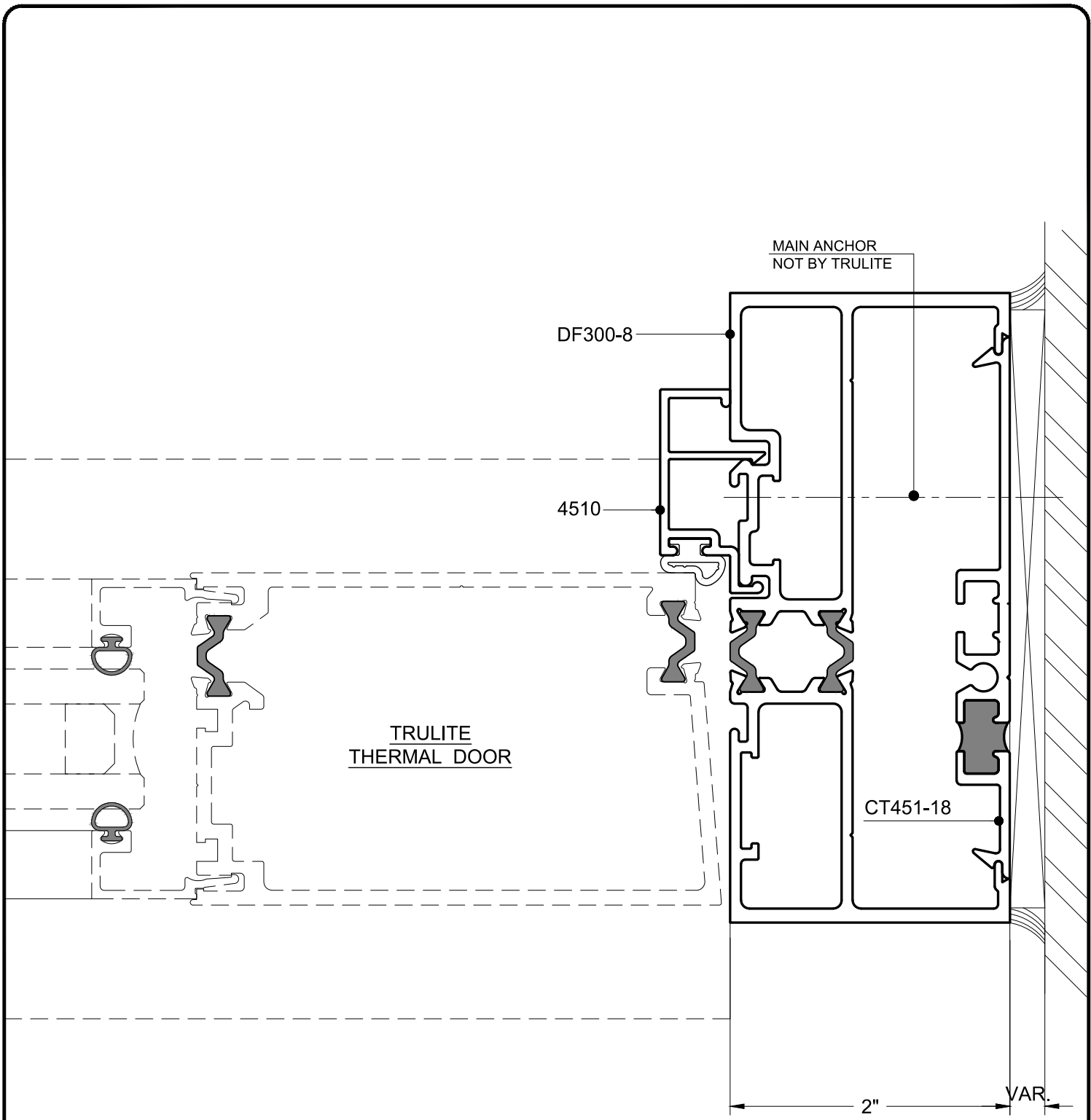
9 THERMAL DOOR JAMB WITHOUT SIDELITE
